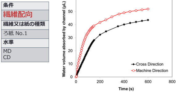
繊維の配向方向と吸水速度の関係
