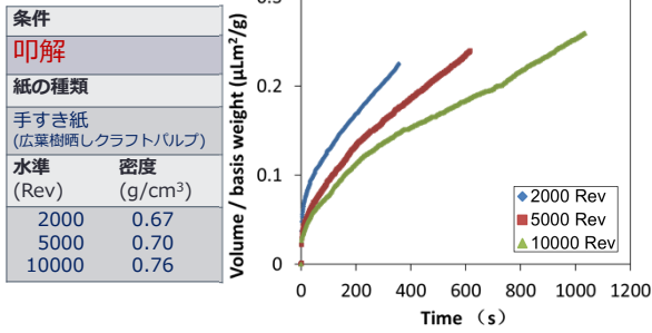
叩解度の異なる試験用手すき紙の吸水速度
