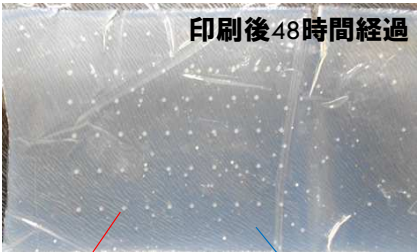
大腸菌のドット
