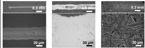
銀配線のSEM画像
