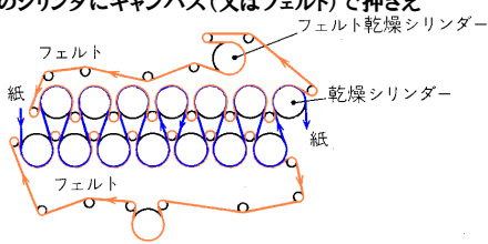
図 4.25 抄紙機ドライヤパート 16)
