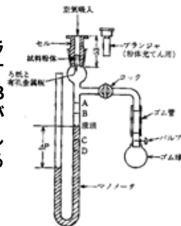
プレーン空気透過装置
