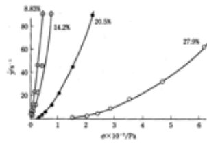
図 1.31 アレーキ系ススペンションの流動曲線
