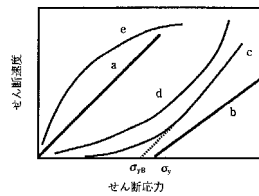
a: ニュートン流動, b: 塑性流動, c: 擬塑性流動, d: 狭義の非ニュートン流動, e: ダイラタント流動の(a,e)は降伏値(ビンガム降伏値)を表す
