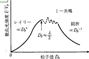
図 2・15 粒子体積当りの散乱光強度の粒子径による変化
