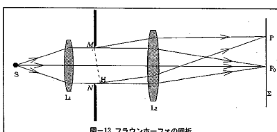
図-13 フラウンホーファの回折
