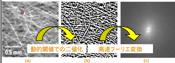
紙表面の光学顕微鏡写真 (a), 二値化画像 (b) 及びパワースペクトル (c)
