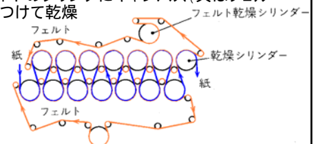
図 4.25 抄紙機ドライヤパート (4)
